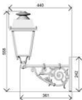
potence PO37 fonte avec lanterne BG1 ref PO37BG1P
